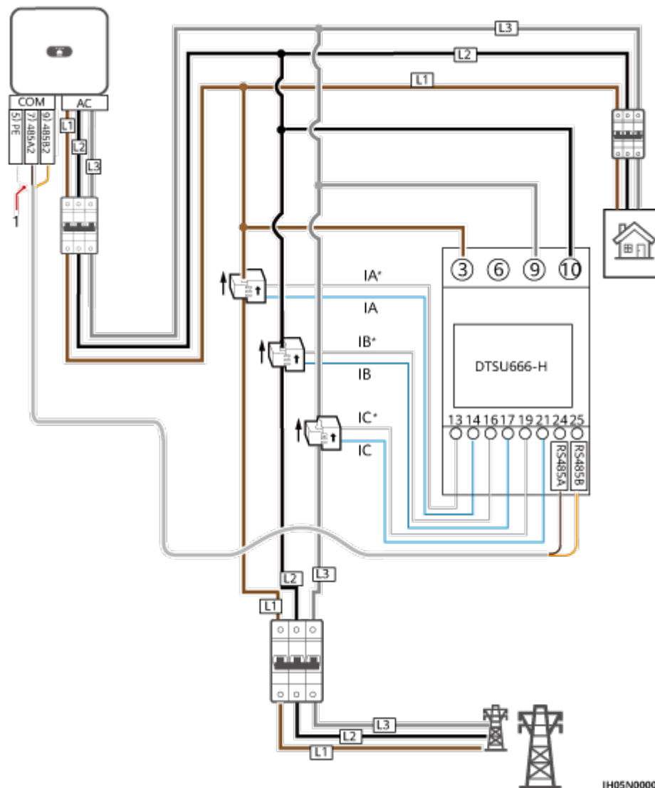
Abbildung 5-22 DTSU666-H dreiphasige dreidrigige Kabelverbindung (Smart Dongle-Vernetzung)
