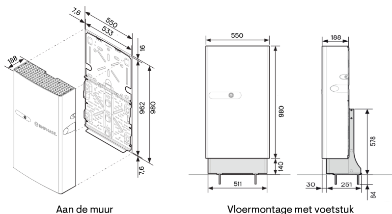
Afmetingen in mm
