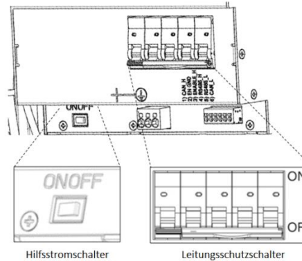
Bild 1: LG RESU Hochvoltbatteriespeicher – Trennvorrichtungen, Sicherungshebel und Hilfsschalter
