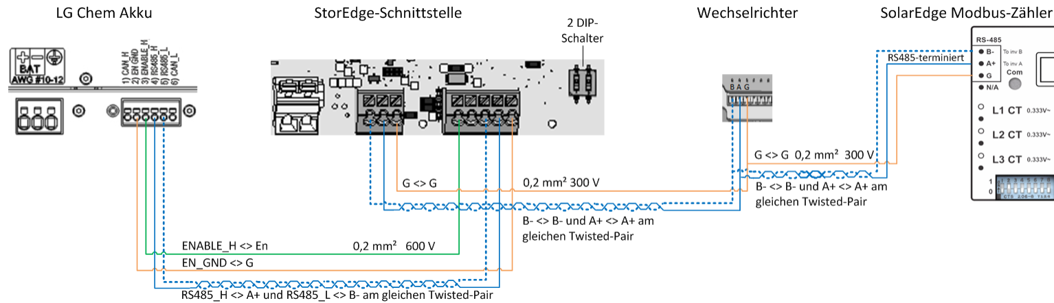
Abbildung 3: Anschluss eines LG Chem RESU7H/10H Hochvoltbatteriespeichers an die SolarEdge StorEdge™ Schnittstelle mit DIP-Schaltern und einem SolarEdge Wechselrichter mit SolarEdge Modbuszähler
