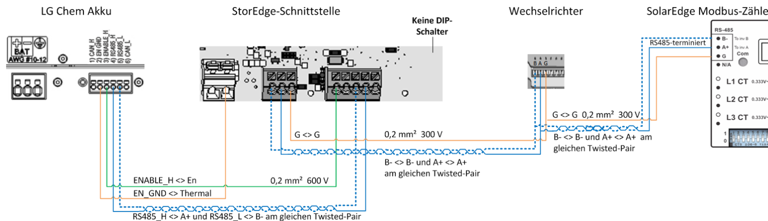
Abbildung 2: Anschluss eines LG Chem RESU7H/10H Hochvoltbatteriespeichers an die SolarEdge StorEdge™ Schnittstelle ohne DIP-Schaltern und einem SolarEdge Wechselrichter mit SolarEdge Modbuszähler
